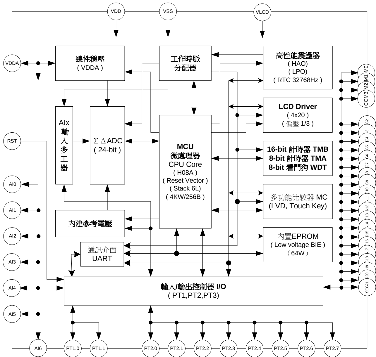
图 3-1 HY13P53B 内部方块图
