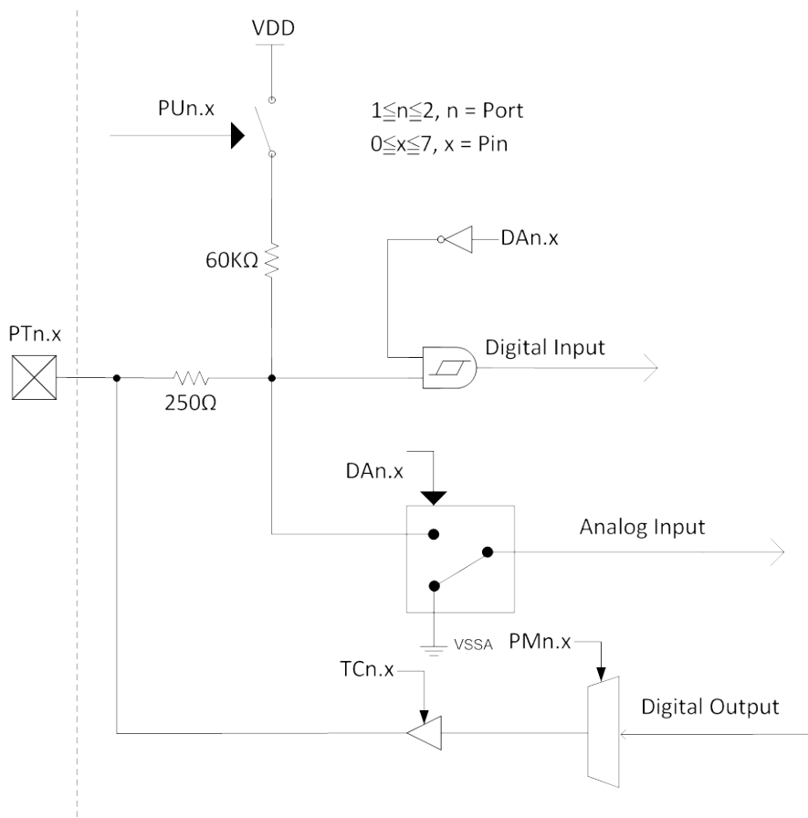
圖 4-9 GPIO 方塊圖
