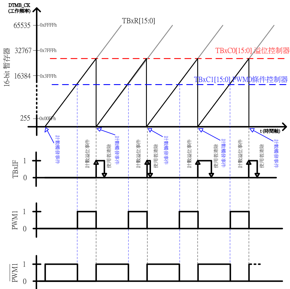
圖 11-6 PWM1O 波形與使用示意圖
