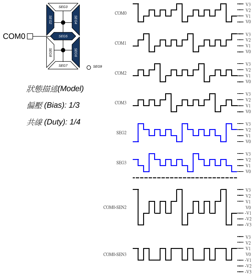
圖 14-3 輸出波形-4 共線
