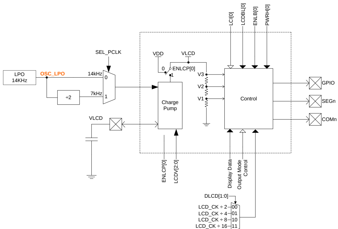
圖 14-1 LCD 方塊圖
