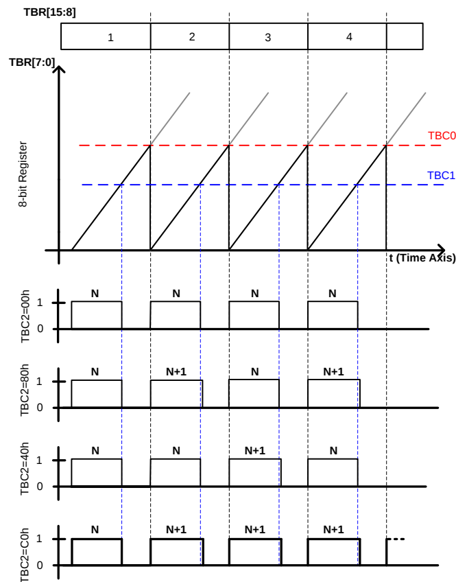
圖 11-10 PWM5O 輸出波形示意圖 1
