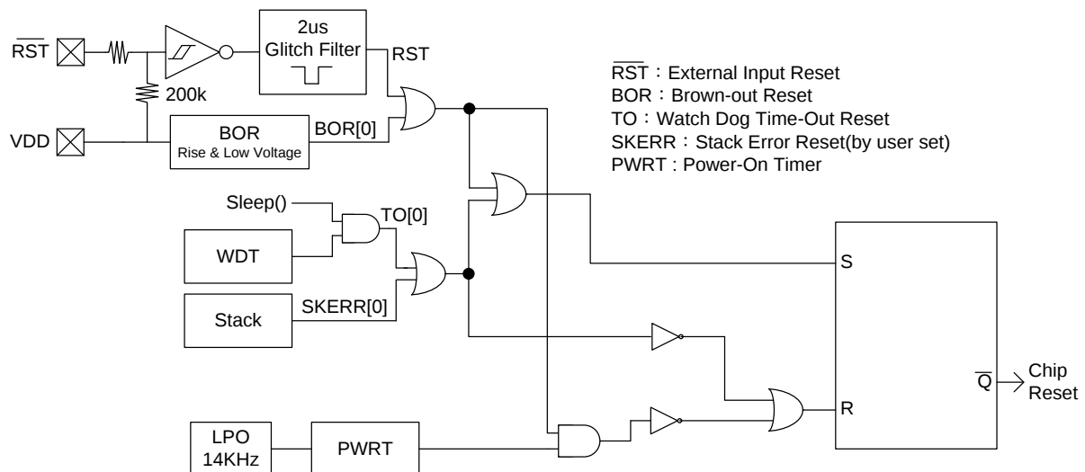
圖 4-1 復位方塊圖
