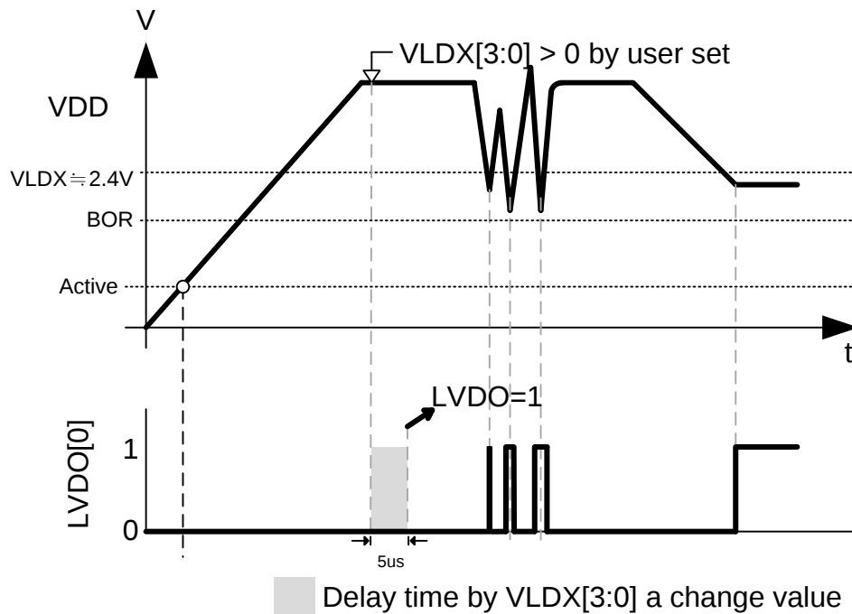
圖 8-2 LVD 時序圖
