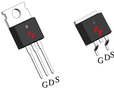
TO-220FB-3L TO-263-2L
