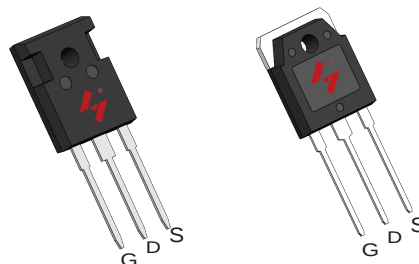
TO-247A-3L
