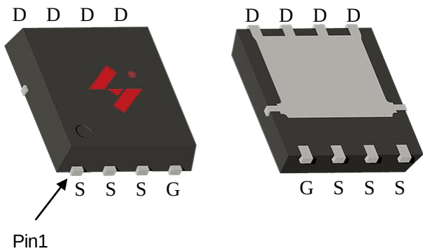
PDFN5*6-8L
