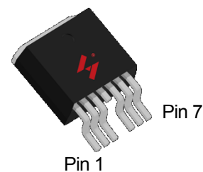
TO-263-6L
