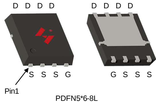
PDFN5*6-8L
