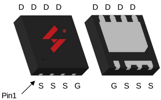
DFN3*3-8L
