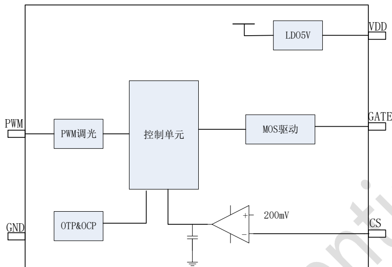
图 7- 1 结构框图
