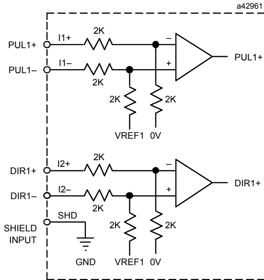
Negative Loop (PUL/DIR Mode)
