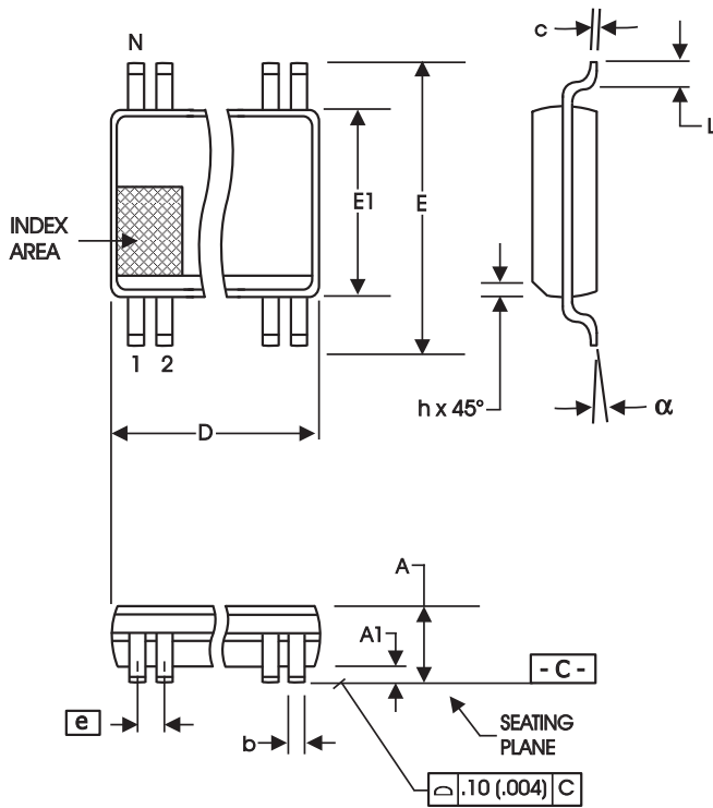
300 mil SSOP
