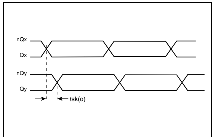
Output Skew
