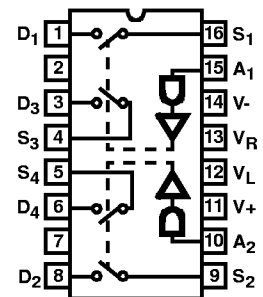
DUAL DPST HI-5045 (50Ω), HI-5049 (25Ω)
