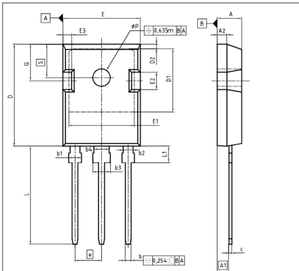
TO247-3
