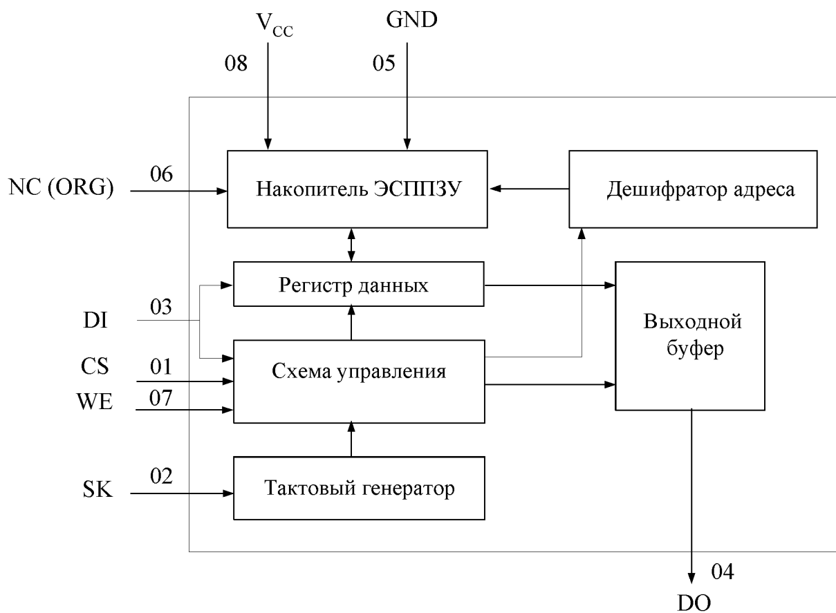
Рисунок 3 – Структурная схема микросхем IN93AA66AN/AD, IN93AA66BN/BD, (IN93AA66CN/CD)
