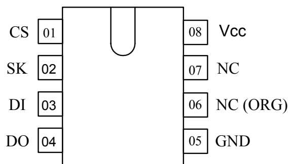
Рисунок 2 – Обозначение выводов в корпусе микросхем IN93AA66AN/AD, IN93AA66BN/BD, (IN93AA66CN/CD)
