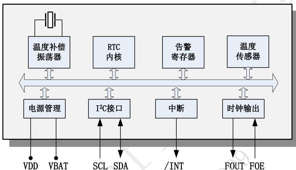
图 1 原理框图
