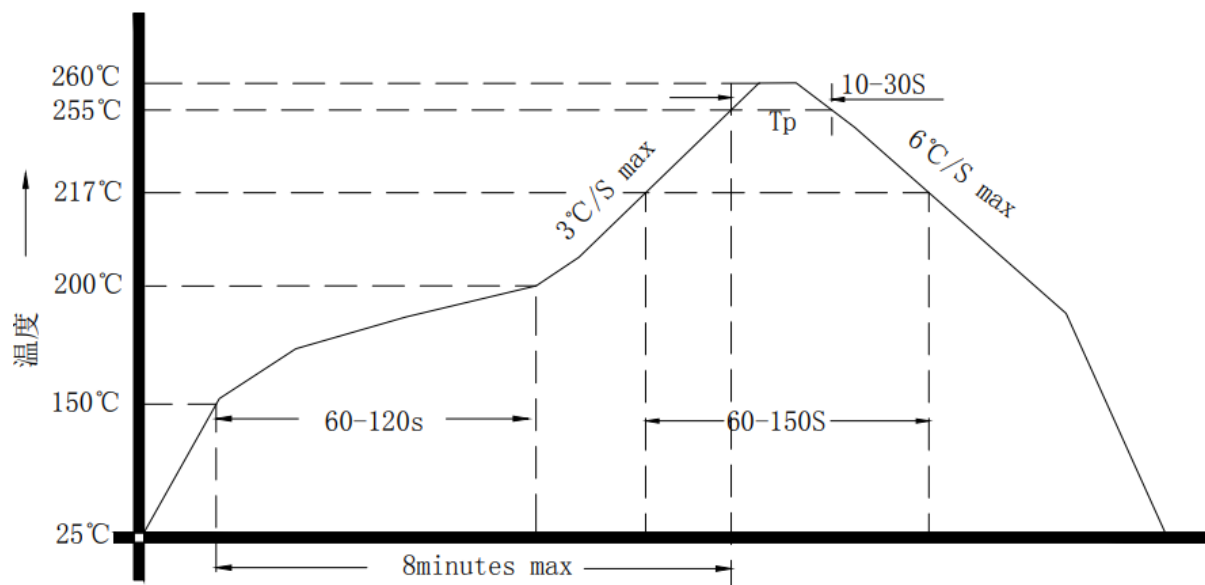
图 10 回流焊曲线
