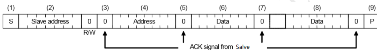
图 6 写序列
