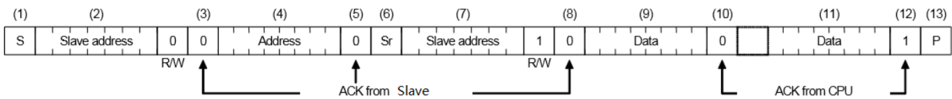
图 7 读序列
