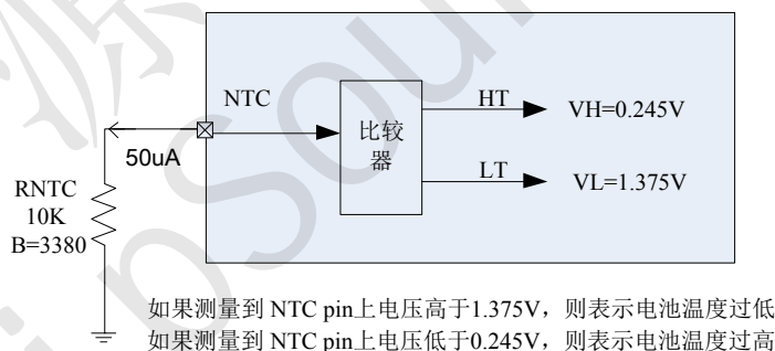
图 7 NTC 框图
