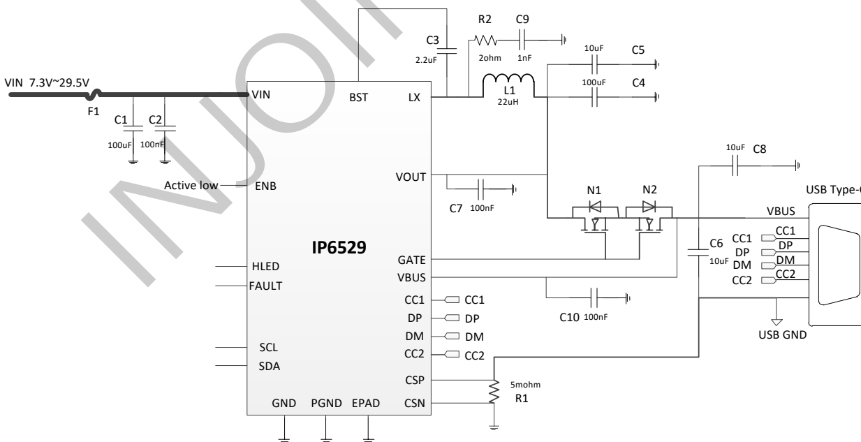
图 9 IP6529_Q1 支持外部采样电阻和路径 MOS 的 PD 快充输出应用原理图
