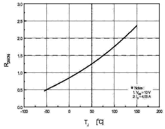
R DS(on) - T J
