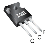
IRG8P40N120KDPbF TO-247AC
