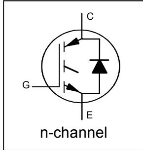
IRG8P60N120KDPbF TO-247AC
