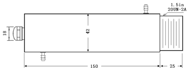
图 5-1b 外型尺寸
