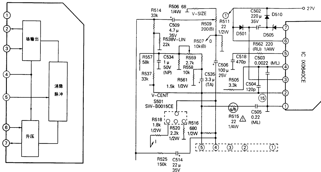
集成电路内部方框图及外部电路图
