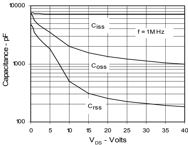
Fig. 11. Capacitance
