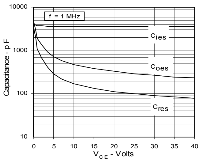
Fig. 15. Capacitance
