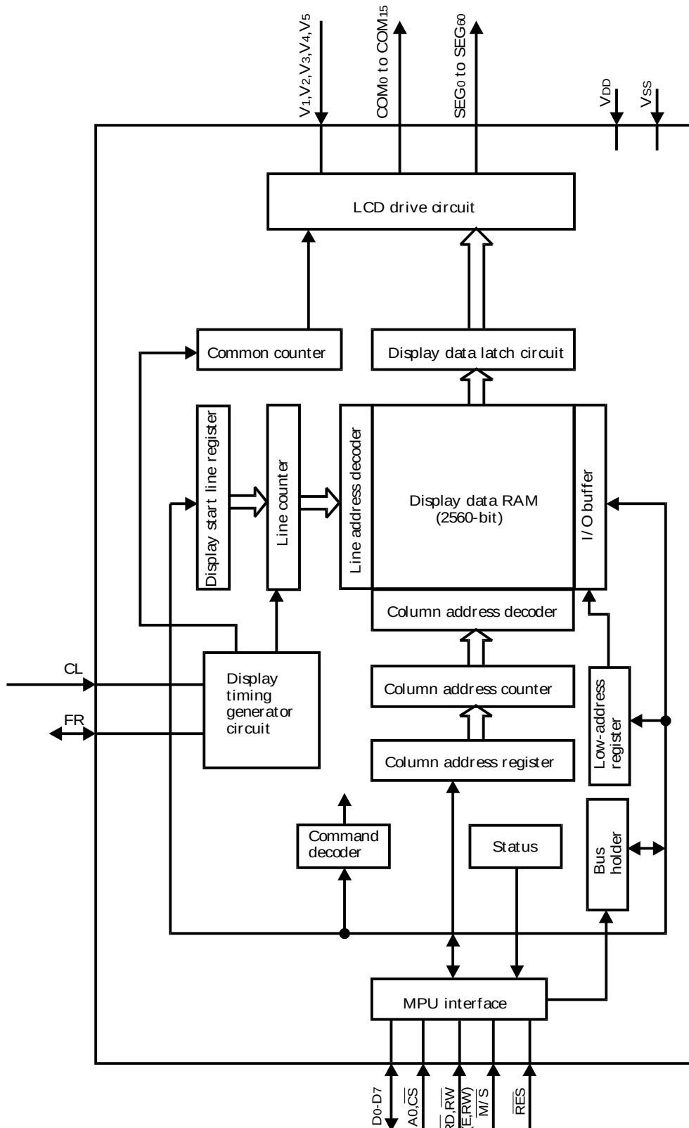
BLOCK DIAGRAM IZD1520AA
