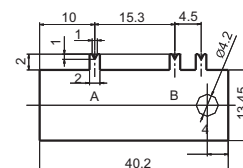
F29( h=1, R=500 ), F30( h=2, R=250 )
