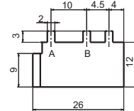
F7( h=1, R=360 ), F8( h=2, R=180 )
