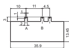
F25( h=1, R=380 ), F26( h=2, R=190 )
