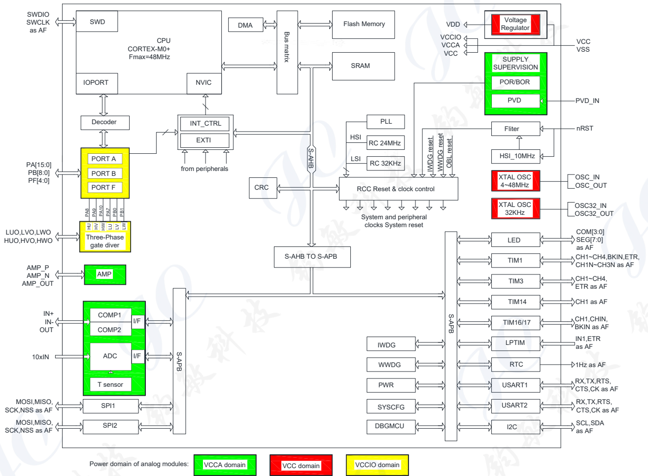
图 1-1 功能模块
