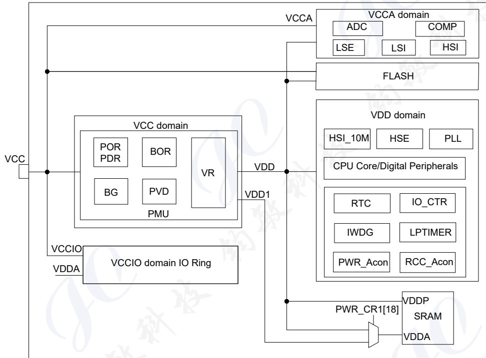
图 2-2 电源框图
