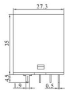
HHC68A-1C(JQX-13F-1C/LY1)
