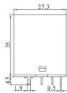
HHC68A-2C(JQX-13F-2C/LY2)
