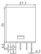
HHC68A-4C(JQX-13F-4C/LY4)
