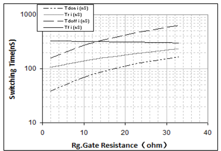
Switching Time vs Rg(175°C) VGE=15V, VCE=600V, IC=75A
