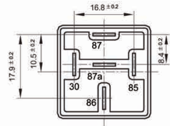
(底视图)
