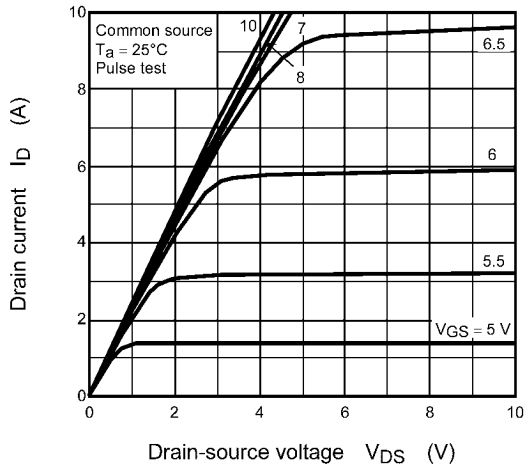
Fig. 8.1 I_D - V_{DS}
