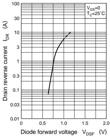
I_{DR} - V_{DSF}
