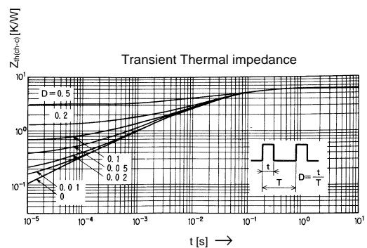
Zth(jc-e)
