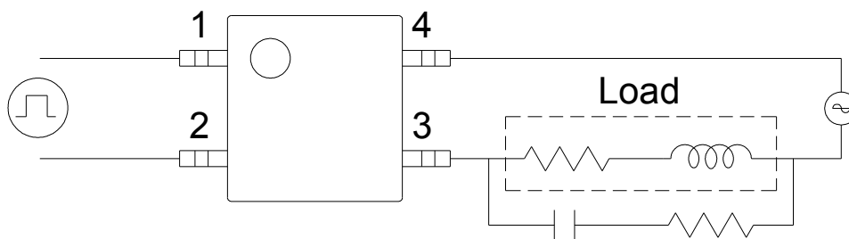
R-C Snubber
