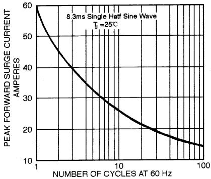
FIG. 1-MAXIMUM NON - REPETTIVE FORWARD SURGE CURRENT - PER ELEMENT
