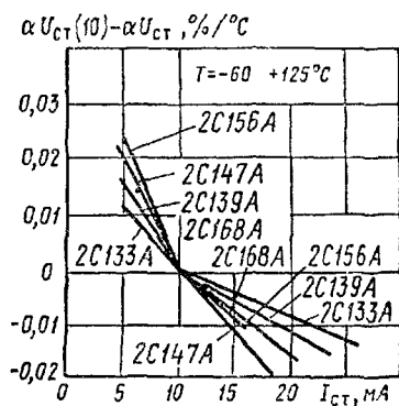
Зависимости температурного коэффициента напряжения ста- билизации от тока
