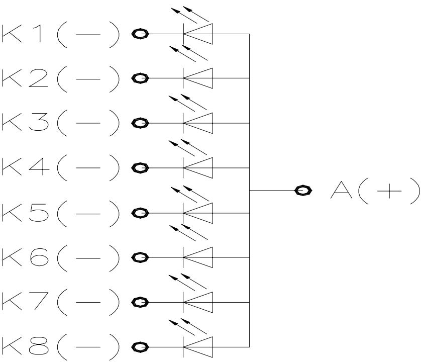
BLU C I R C U I T D I A G R A M
