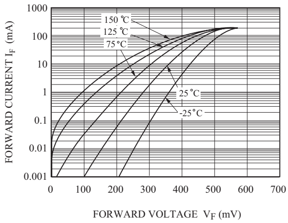
I_F - V_F
