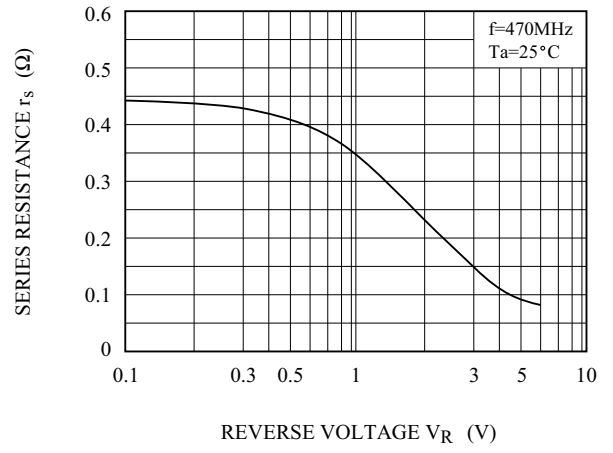
r_s - V_R
