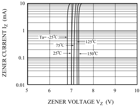
V_Z - I_Z
