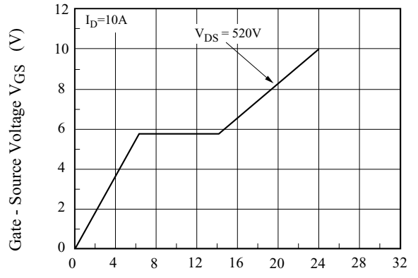
Fig8. Q_g - V_{GS}
