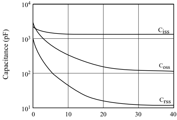
Fig 7. C - V_{DS}
