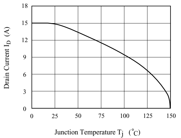
Fig10. I_D - T_j
