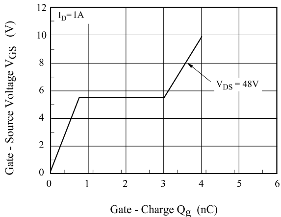
Fig8. V GS - Q g
