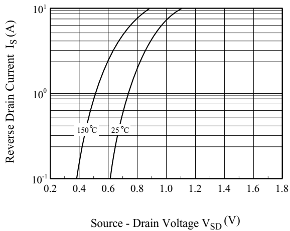
I_S - V_{SD}
