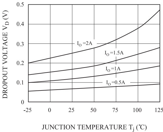
Fig. 7 T_j - V_D
