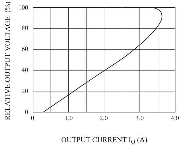
Fig. 4 I_O - V_O
