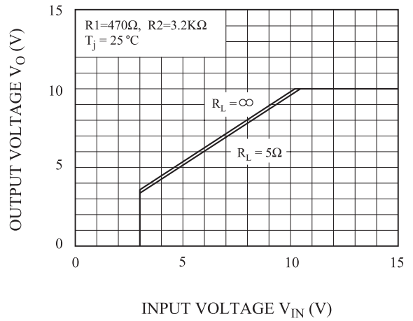
Fig. 6 V_{IN} - V_{OUT}
