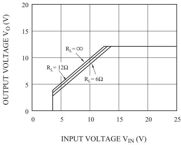
Fig.10 V_{IN} - V_O (KIA278R12)
