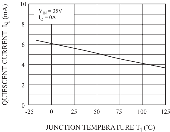
Fig. 8 I_q - T_j
