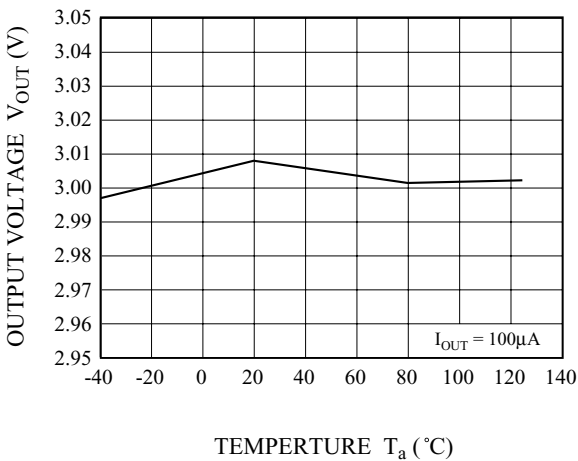
Fig. 5 T a - V OUT
